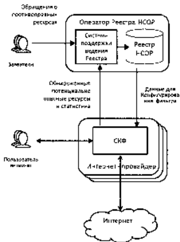
Рисунок 6. Принцип контроля доступа через Реестр NSRP
